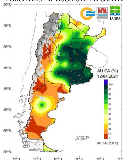
PORCENTAJE DE AGUA ÚTIL EN CAPA ARABLE
