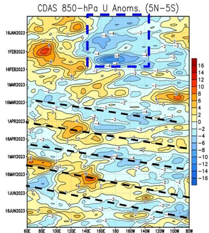
Figura 6 - Anomalías de viento zonal promediado en la región 5°S-5°N del 01 de enero al 02 de julio de 2023 - Fuente: Climate Prediction Center (CPC)-NOAA
