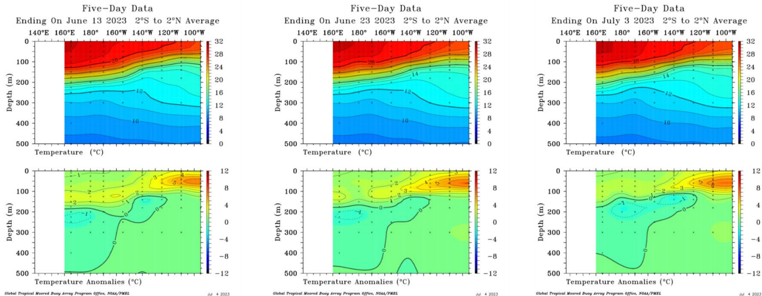
Figura 4 – Corte profundidad vs. longitud de la temperatura del agua del mar y su anomalía en el Pacífico ecuatorial, correspondiente al promedio pentádico que termina el 13 de junio (izquierda), el 23 de junio (centro) y el 03 de julio de 2023 (derecha). Fuente: Pacific Maritime Environmental Laboratory (PMEL)-NOAA
