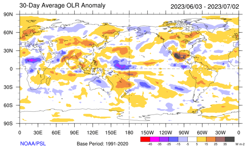
Figura 8 – Anomalías de radiación de onda larga saliente (OLR) del 03 de junio al 02 de julio de 2023 - Fuente: NOAA-CIRES/CDC
