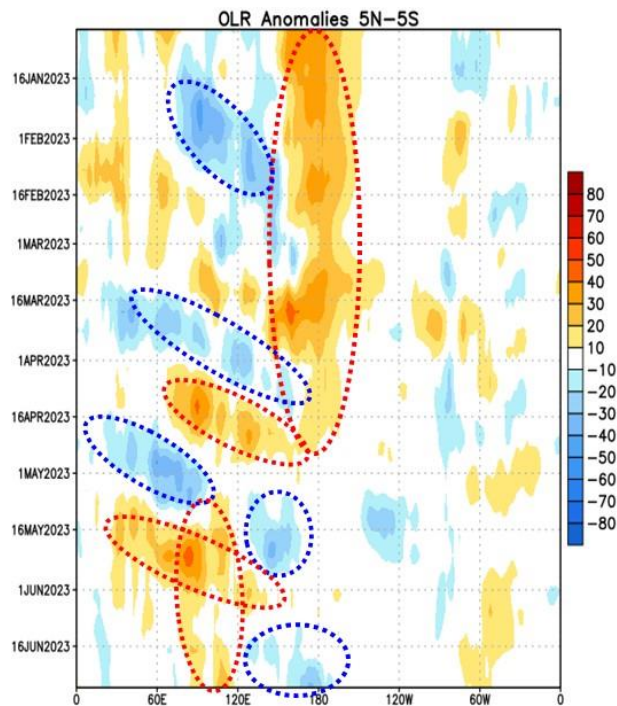
Figura 7 – Anomalías de radiación de onda larga saliente (OLR) promedio en la región 5°S-5°N, del 01 de enero al 02 de julio de 2023 - Fuente: Climate Prediction Center (CPC)-NOAA
